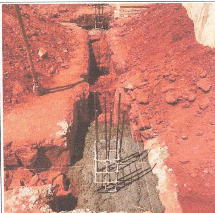
Descrição: ARMAÇÃO E CONCRETAGEM DOS BLOCOS
