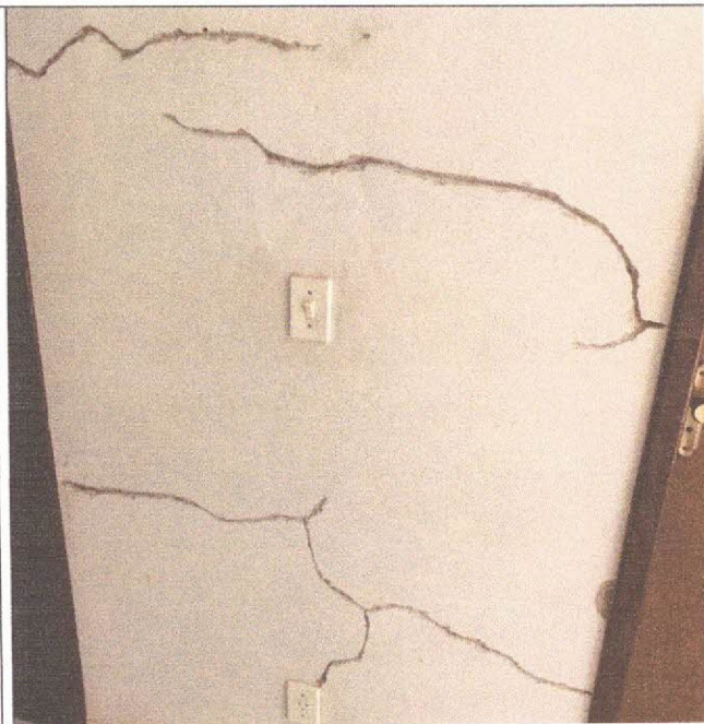
Descrição: PREPARATIVO PARA SELAMENTO DAS TRINCAS
