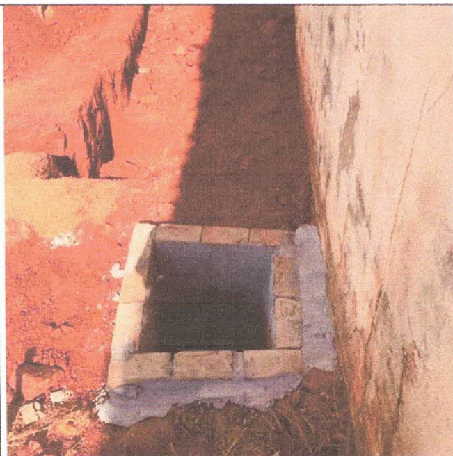
Descrição: CAIXA DE PASSAGEM EM ALVENARIA
