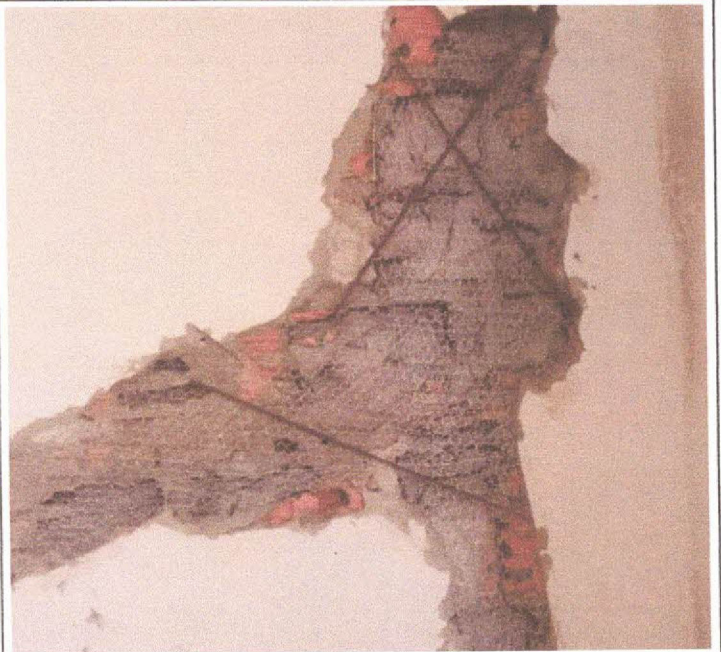
Descrição: REPARO DAS TRINCAS COM GRAMPOS E TELAS
