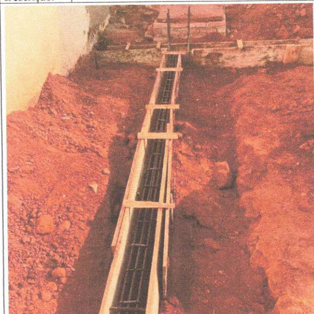
Descrição: MONTAGEM DE FORMAS PARA VIGAS BALDRAMES
