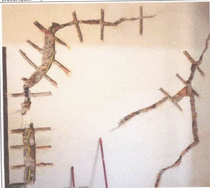
Descrição: REPAROS DE TRINCAS COM GRAMPOS E TELAS
