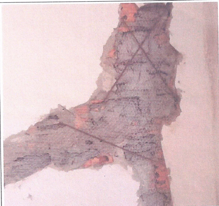
Descrição: REPARO DAS TRINCAS COM GRAMPOS E TELAS
